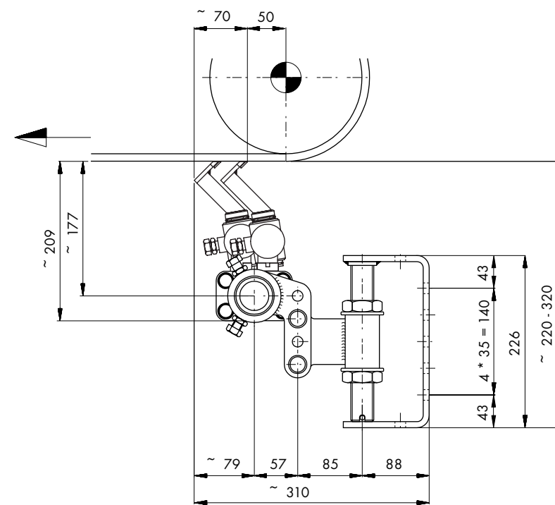
Położenie modułów skrobaka przed napięciem
