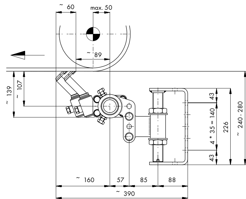
Widok skrobaka przed dociśnięciem do taśmy
