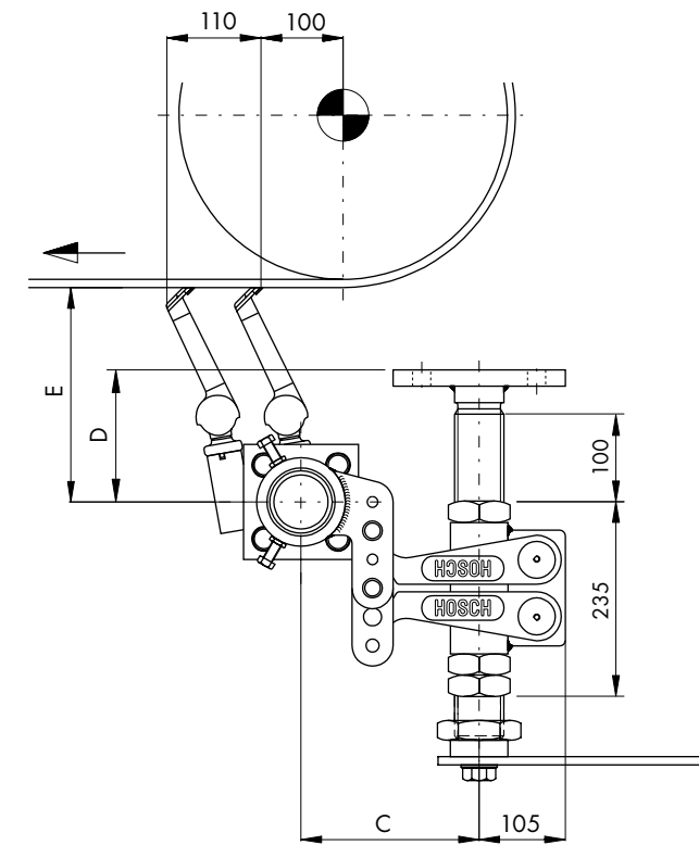
Widok skrobaka przed dociśnięciem do taśmy
